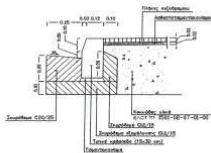
Εικόνα 7.1: Τυπική διαμόρφωση ρείθρου-κράσπεδου-πεζοδρομίου στις περιοχές παρέμβασης
