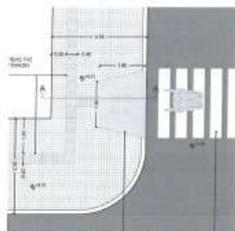
Εικόνα 5.1: Ενδεικτική Διαμόρφωση Διάβσης Πεζών με Ρόμπες
