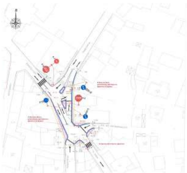
ΣΧΕΔΙΟ Σ.3: ΙΣΟΠΕΔΟΣ ΚΟΜΒΟΙ ΣΙΜΟΠΟΥΛΟΥ – ΠΛΑΝΟΥΡΓΙΑ – ΠΑΠΑΘΑΝΑΣΙΟΥ – ΣΑΘΑ
